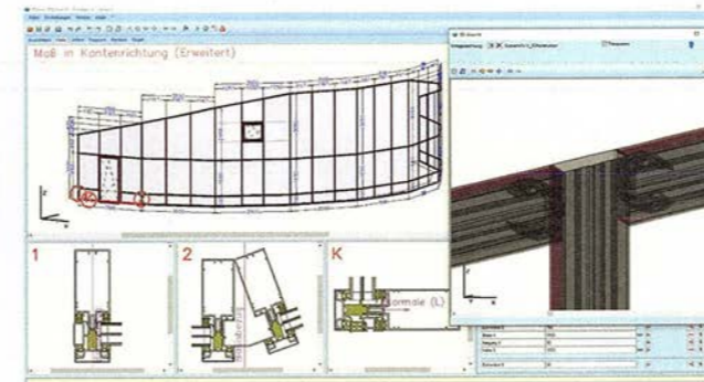
/ Neben Fassaden und Wintergärten können mit Klaes 3D auch freistehende Pergola-Systeme, Vordächer u. v. m. konstruiert, kalkuliert und produziert werden.
